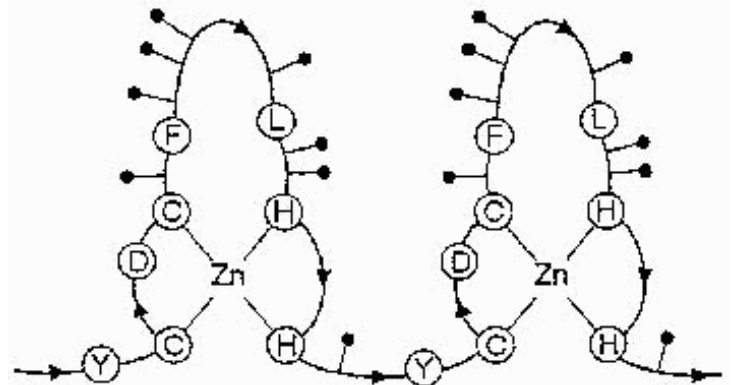
Figura 9. Estructura de los dedos de zinc de una proteína intercalante del ADN (según Miller)
